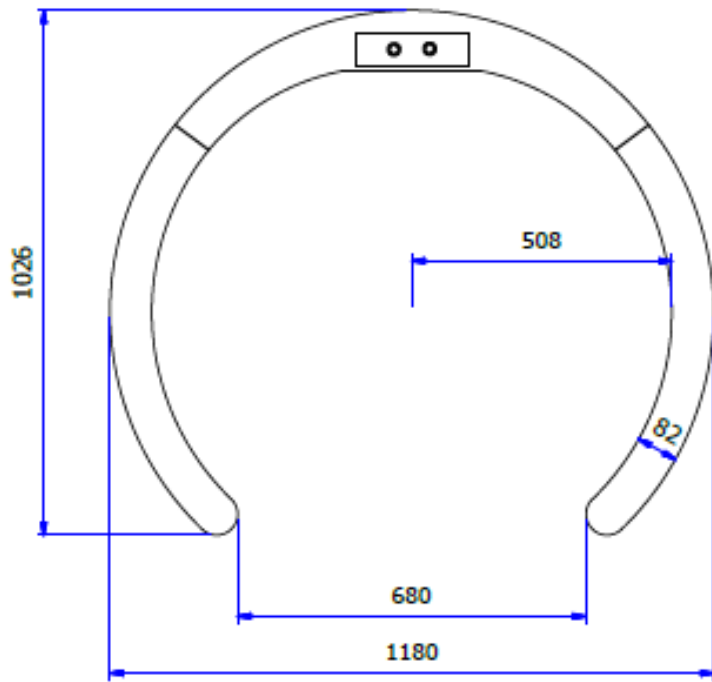
PLAN (1180 W x 1026 L x 2170 H)
